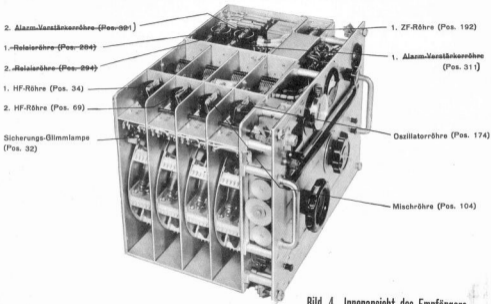
Bild 4. Innenansicht des Empfängers (von oben links)
